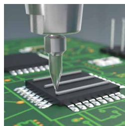
集積回路に 放熱グリースを 線塗布
